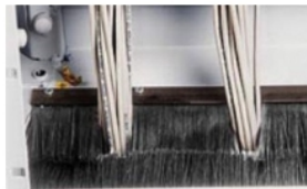
Przepust szczotkowy dachowy do...
